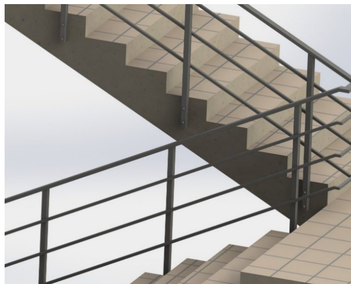
Поручень 50x25мм , стойка 40x40мм , ригель 20x20мм.
